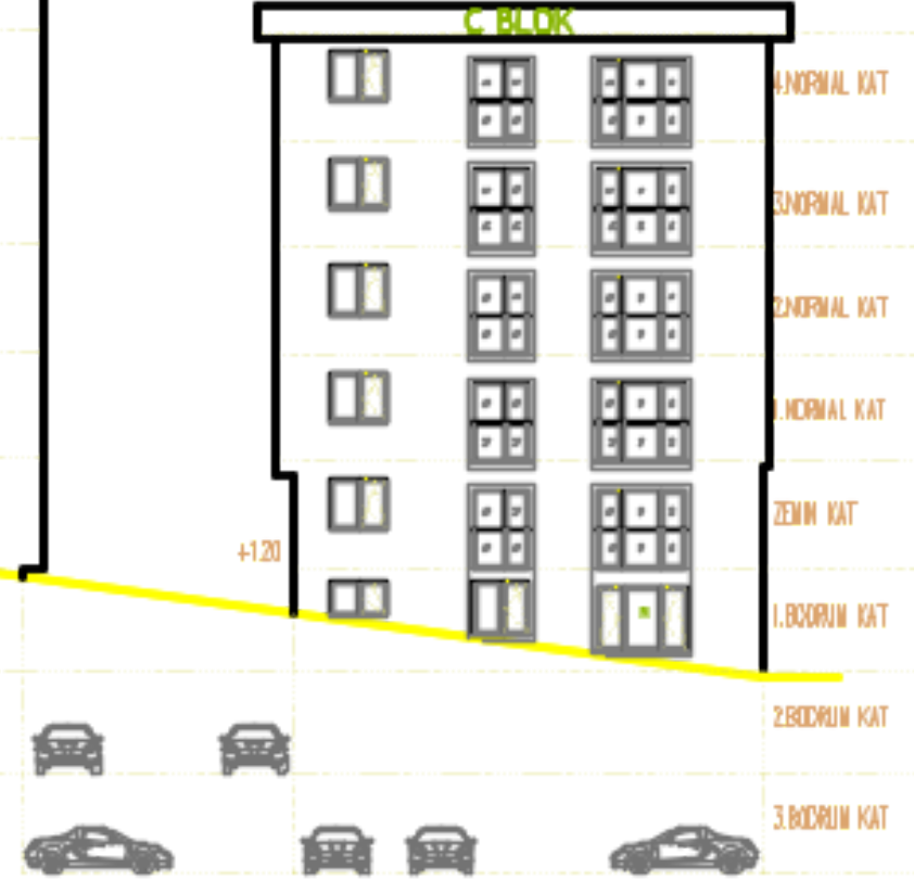
(C BLOK) SOL YAN GÖRÜNÜŞ - ÖLÇEK:1/50
