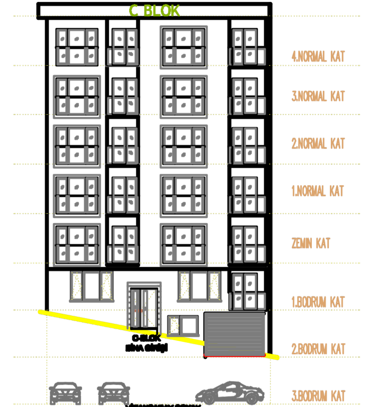
(C BLOK) ÖN GÖRÜNÜŞ - ÖLÇEK:1/50
